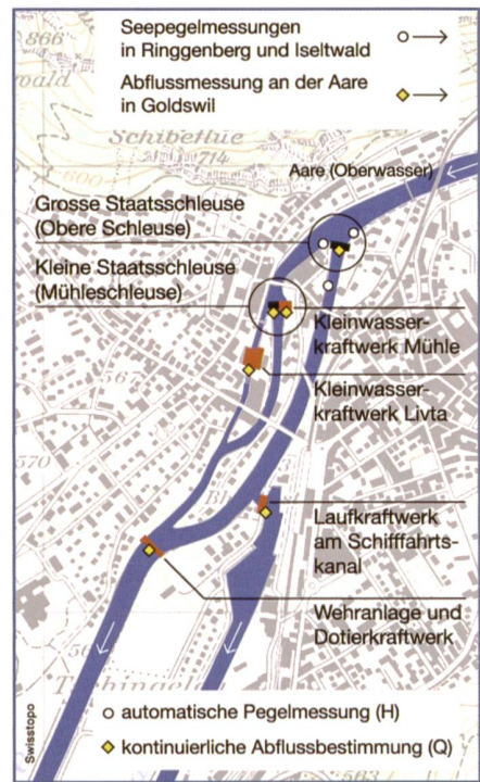
Bild 3. Lage und Art der Abflussorgane und der Messeinrichtungen (Quelle [1]).
