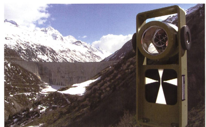
Bild 9. Präzisionsreflektoren für die Distanzmessung mit dem Mekometer ME5000.
