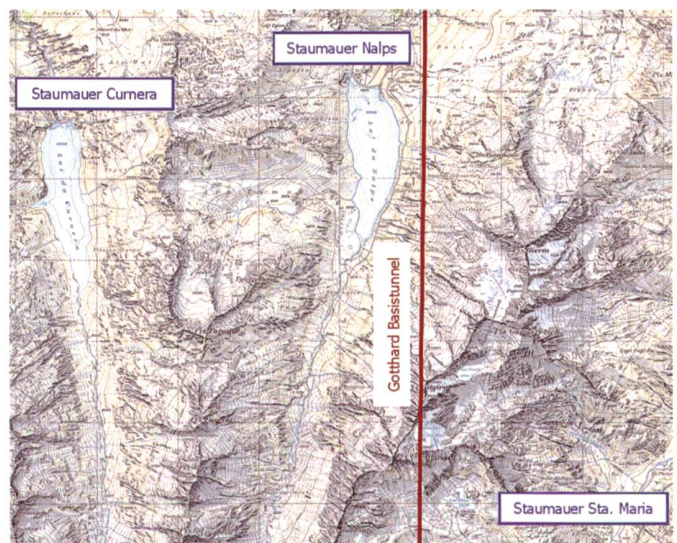
Bild 1*. Übersicht Linienführung Gotthard-Basistunnel.
