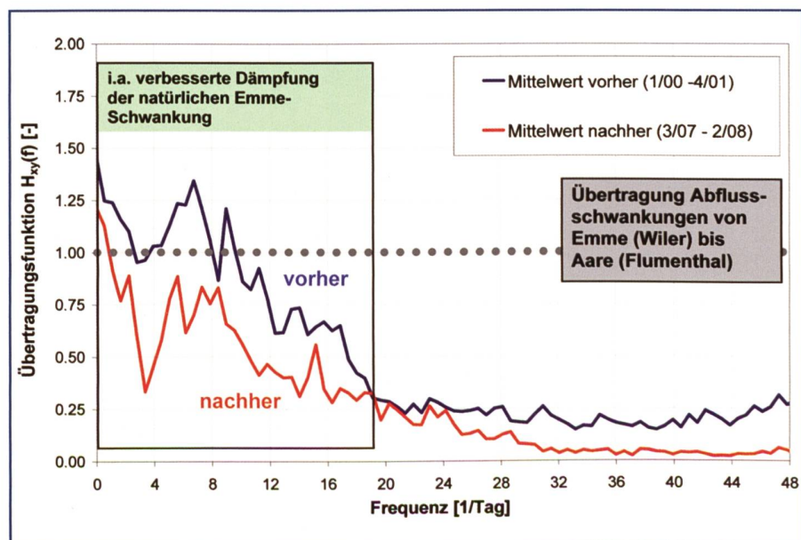
Bild 6. Übertragungsfunktionen vom Pegel Brügg-Ägerten zum Pegel Brugg vor bzw. nach Modifikation der Regelungen.
