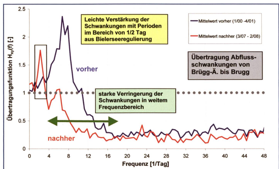
Bild 5. Übertragungsfunktionen vom Pegel Brügg-Ägerten zum Pegel Brugg vor bzw. nach Modifikation der Regelungen.
