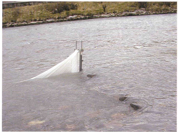
Bild 2. Driftversuche in der Aare im März/April 2008 (Limnex 2009). Links, Messung in unzugänglicher Kanalstrecke mittels Lastwagenkran, Tauchpumpe, Schläuchen, Netz und Bottich; rechts, Messung der Drift mit fixiertem Netz in der Kiesbankstrecke. Fotos Peter Baumann, Limnex AG.
