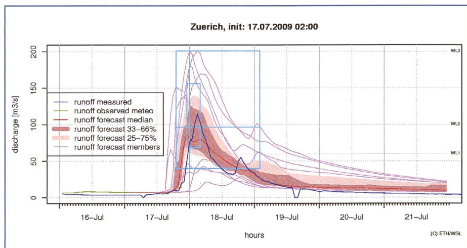
Bild 6. Das Abflussereignis vom 17./18. Juli 2009. Vorhersagen des Modellsystems PREVAH/FLORES für den Abfluss der Sihl beim Hauptbahnhof rund 36 Stunden (Prognose vom 16. Juli; Grafik oben) und zwölf Stunden (Prognose vom 17. Juli; Grafik unten) vor dem Beginn des Ereignisses. Meteorologische Datengrundlage COSMO-LEPS. Die beobachteten Abflüsse (Stundenmittel, blaue Linie) wurden zu Auswertungszwecken nachträglich jeweils für den gesamten dargestellten Zeitraum angegeben; in der Abflussprognose endet sie zum Zeitpunkt der Modellrechnung (vgl. Bild 4).
