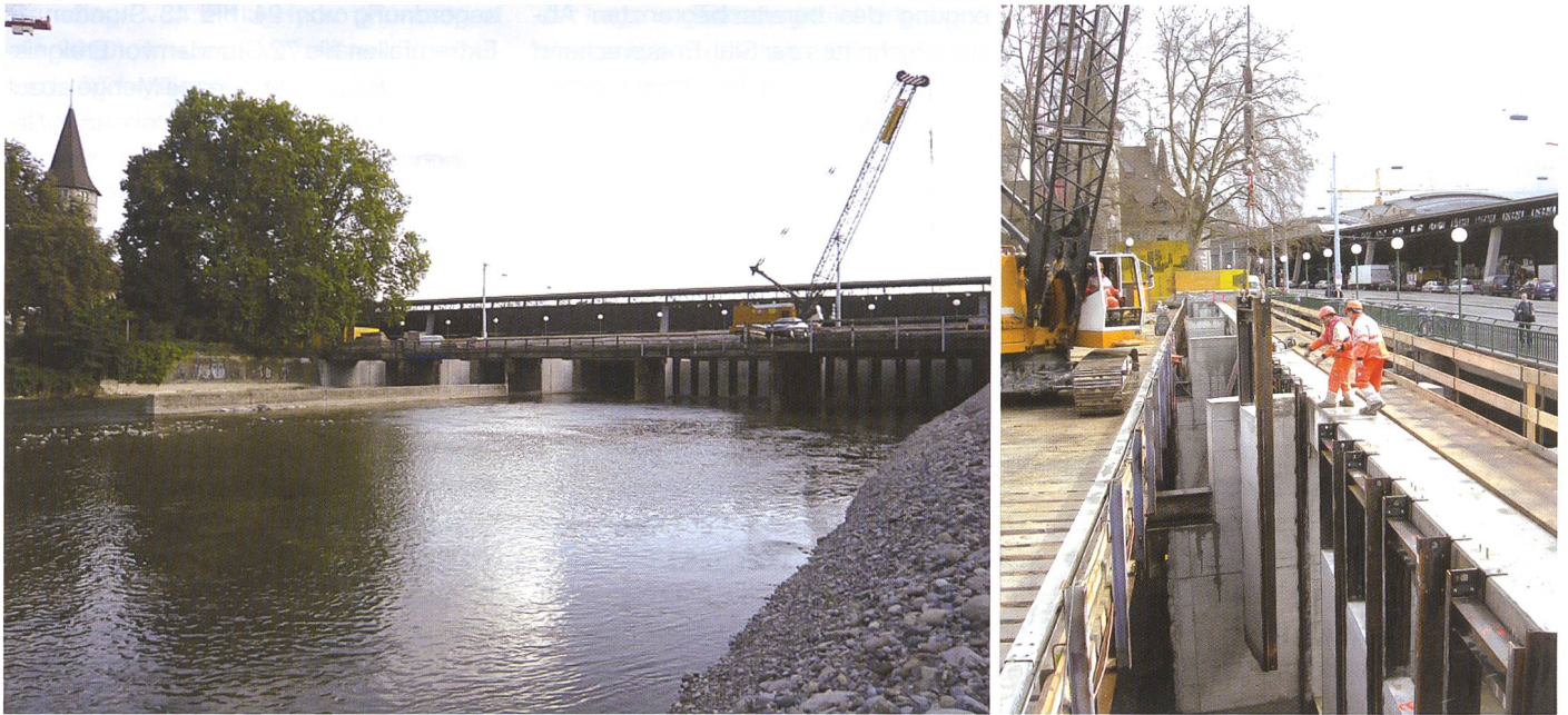
Bild 5. Fluttore unterstrom (links): Spundwandbohlen im Wechsel mit Betonelementen. Im Rahmen einer Baustellenflutung werden diese Elemente mittels Seilbagger hochgezogen (rechts) (Quelle: igzalo).
