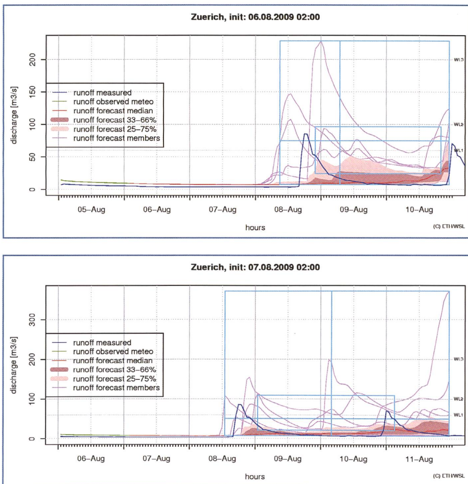
Bild 7. Das Abflussereignis vom 8./9. August 2009. Vorhersagen des Modellsystems PREVAH/FLORES für den Abfluss der Sihl beim Hauptbahnhof rund 60 Stunden (Prognose vom 6. August; Grafik oben) und 36 Stunden (Prognose vom 7. August; Grafik unten) vor dem Beginn des Ereignisses. Meteorologische Datengrundlage COSMO-LEPS. Die beobachteten Abflüsse (Stundenmittel, blaue Linie) wurden zu Auswertungszwecken nachträglich jeweils für den gesamten dargestellten Zeitraum angegeben; in der Abflussprognose endet sie zum Zeitpunkt der Modellrechnung (vgl. Bild 4).
