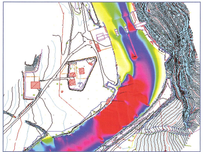
Figure 5. Vitesses d'écoulement au droit du barrage pour un débit de 1270 m 3 /s dans la géométrie «après purge» (couleur jaune: 1 m/s, couleur rouge: 6 m/s).
