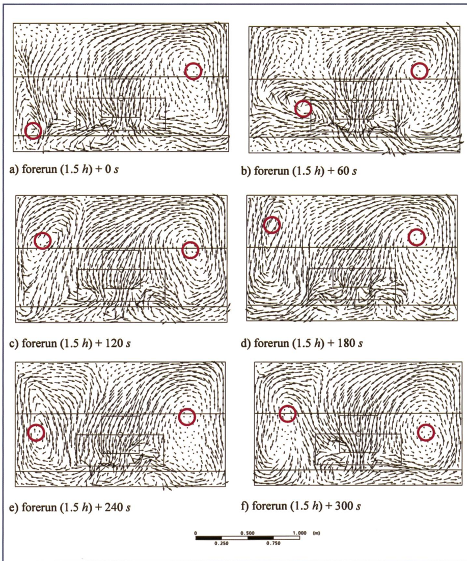
Bild 9. Zeitsequenz des numerisch simulierten Strömungsbildes in der Querebene ( C/B = 0.175 , h_f/B = 0.25 ). Von a) bis f): Instationärer Vorlauf (1.5 h) + 0 s, 60 s, 120 s, 180 s, 240 s, 300 s. Die Wasserfassung ist durch den kleinen Kreis angegeben. Die Rotationszellen sind durch die grösseren roten Kreise gekennzeichnet.
