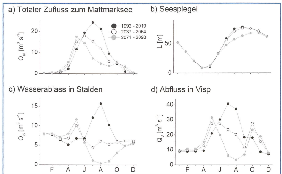
Bild 2. Die wahrscheinlichsten Prognosen der Wasserressourcen im Vispental für die Situation heute (1992–2019; schwarze Punkte), mittelfristige Prognose (2037–2064; weisse Punkte) und langfristige Prognose (2071–2098; graue Punkte).
