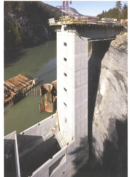
Bild 3. Einlaufbauwerk zum Umleitstollen (EWZ).
