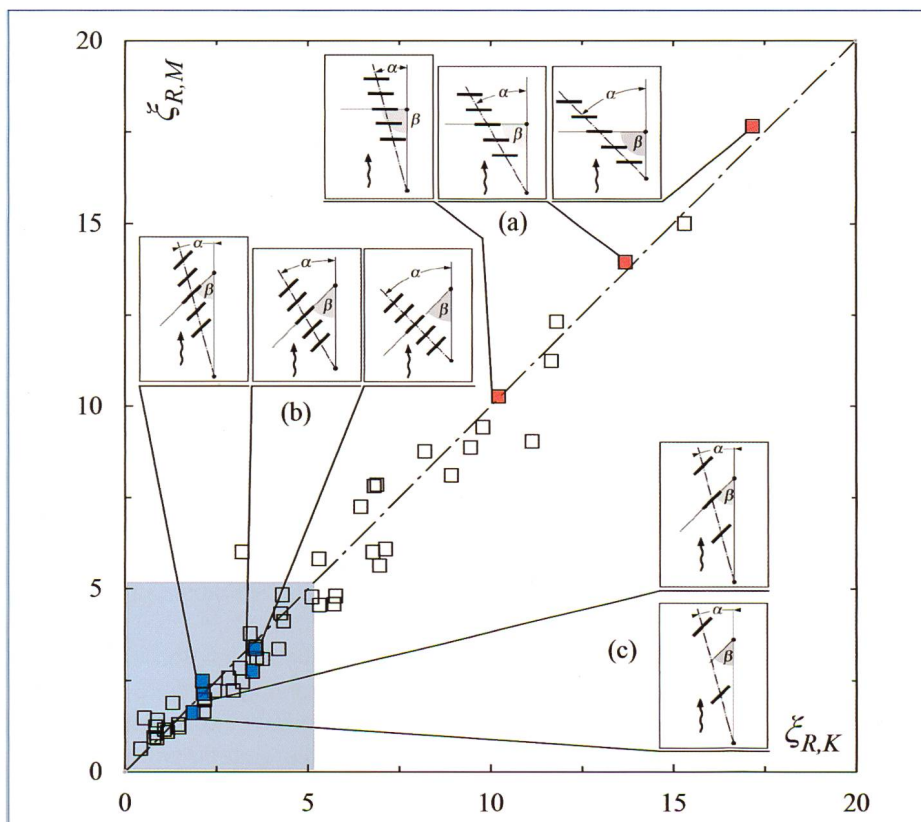
Bild 5. Ergebnisübersicht mit Auswahl wichtiger Leitreechenkonfigurationen: (a) Louver mit \alpha = 15^\circ, 30^\circ, 45^\circ bei B = 6 \text{ cm} ( \sigma = 0.17 ); (b) modifizierte Bar-Racks analog zu (a); (c) modifizierte Bar-Racks mit \alpha = 15^\circ und B = 12 \text{ cm} und 24 \text{ cm} ( \sigma = 0.08 resp. 0.04 ); die blaue Zone repräsentiert Verlustbeiwerte von Einlaufrechen Schweizer Kraftwerke nach Meussurger (2002).
