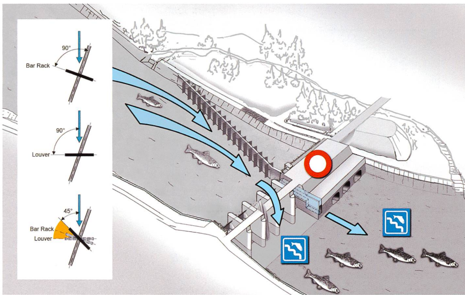
Bild 1. Projektidee mit Einsatz vertikaler Leitreechen und Detailansicht von Louver-, Bar-Rack- und modifizierten Bar-Rack-Systemen.
