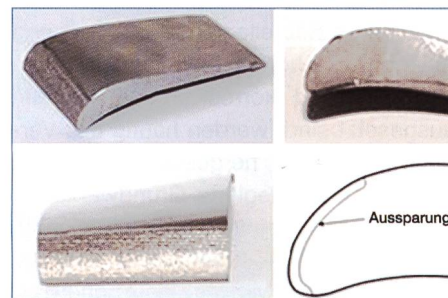
Bild 6. Segment einer Dampfturbinschaufel mit Stellite-Schutzschicht gegen Wassertröpfchenerosion an der Schaufelvorderkante.
