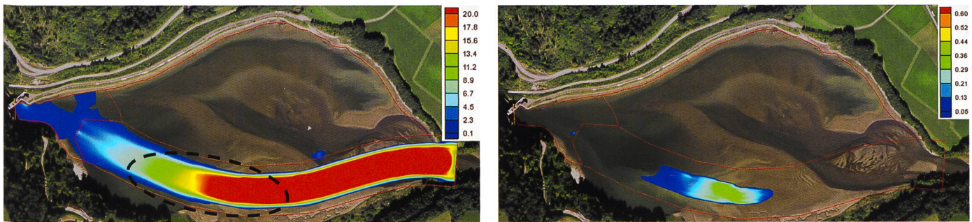
Figure 10. Contrainte de cisaillement et dépôts pour une crue annuelle (100 m 3 /s avec le lac à 860 m s.m.).
