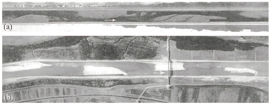
Bild 6. Ähnliche Flussstrecken (a) im geraden Modellkanal, (b) Rhein-Strecke mit Brücke Kriessern-Mädel (Meyer-Peter et al. 1935).
