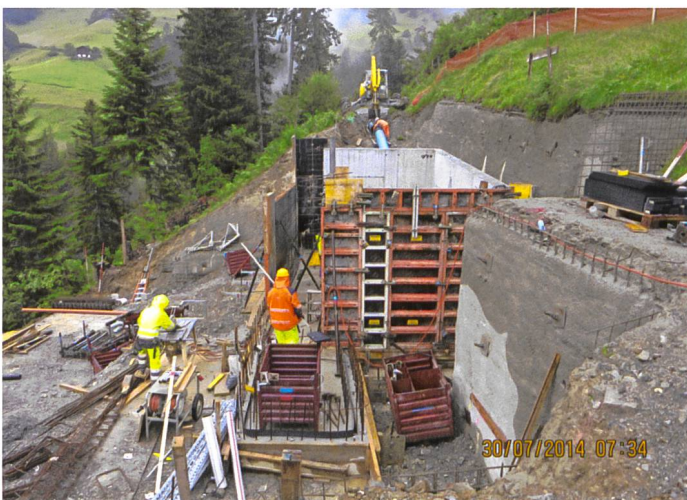
Bild 13. Bau der unterirdischen Zentrale Albrist mit Zusammenschluss Druckleitung im Hintergrund (Juli 2014).
