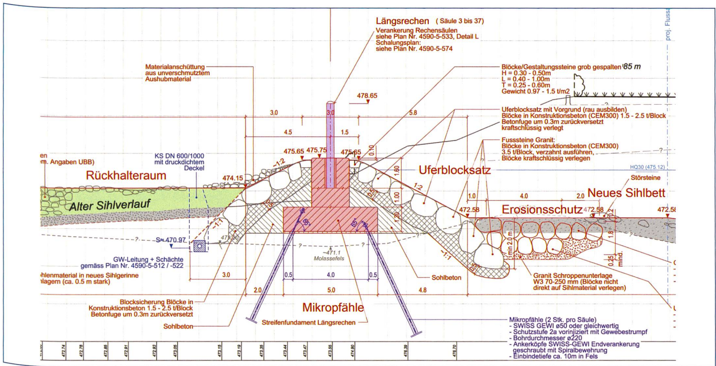
Bild 12. Querschnitt beim Längsrechen: Die Rechenstäbe stehen auf einem Leitdamm. Dieser Damm bewirkt, dass die Abflusstiefe bis zum unteren Ende des Holzrückhalts genügend gross ist, damit dieser von unten her aufgefüllt wird. Das Streifenfundament der Rechenstäbe ist auf zwei Mikropfähle (Zug- und Druckpfahl) pro Rechenstab abgestützt.
