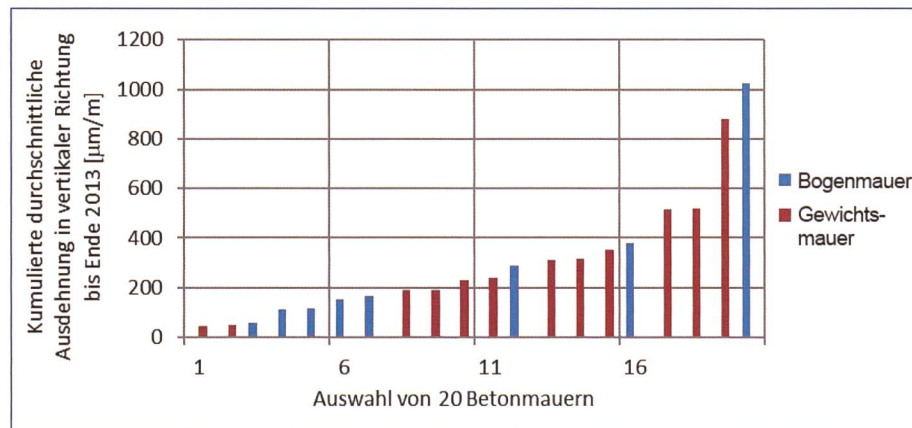
Bild 12. Über die Zeit kumulierte vertikale Ausdehnung der ganzen Mauerhöhe von 20 Talsperren.
