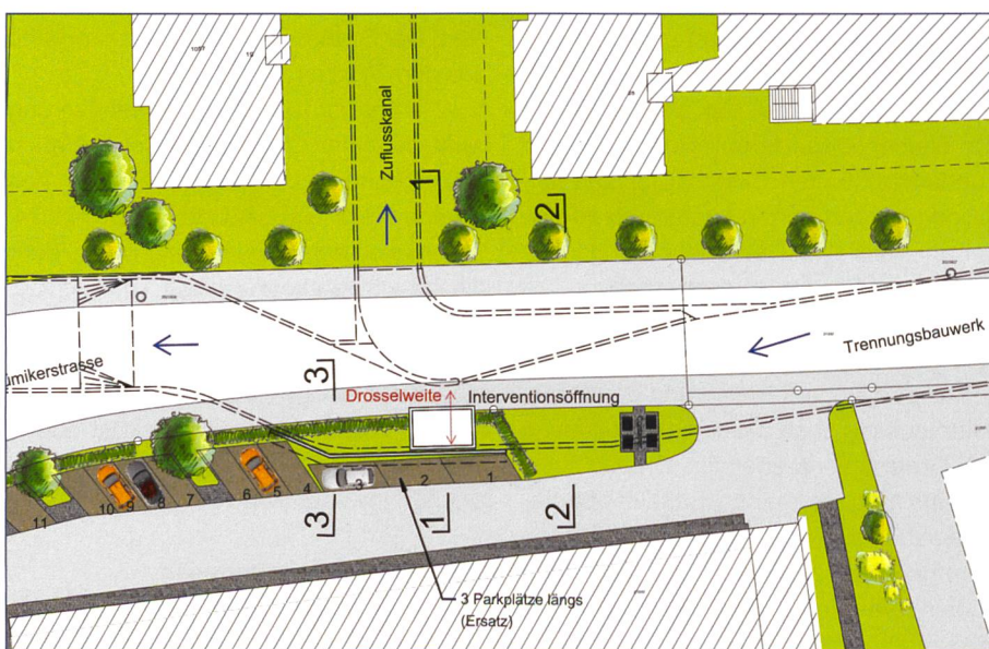
Bild 9. Verschwenkung des Trennungsbauwerks aus der Achse des bestehenden Hochwasserkanals.
