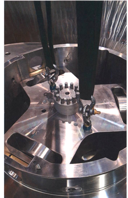
Bild 13: Verstellmechanismus des Kaplan-Laufrades (Foto: Groupe E).
