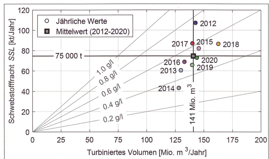
Bild 6: Jährlich turbinierter Schwebstofffrachten in Funktion der entsprechenden Wasservolumina im KW Fieschertal (Betriebsdaten: gkw).
