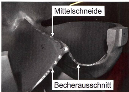
Bild 10: Abgenutzter Becher eines beschichteten Peltonlaufrads (Foto: VAW).
