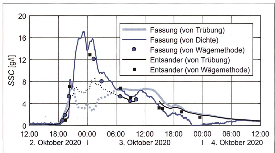
Bild 9: Schwebstofftransport-Ereignis von anfangs Oktober 2020: Schwebstoffkonzentrationen SSC bei den Fassungsbauwerken, die mit mehreren Methoden gemessen wurden (ungültige Messwerte von überlasteten Trübungssonden strichliert).
