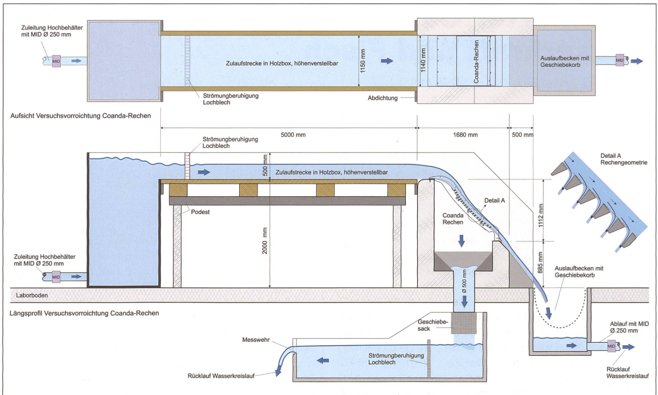
Bild 1: Versuchsvorrichtung.
