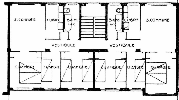
Grundrisse Gruppe A und Gruppe F (Architekt M. Braillard)
