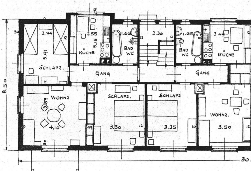
Gemeinnützige Bau- und Wohngenossenschaft „Freistatt“, Thun Wohnungsgrundriß
