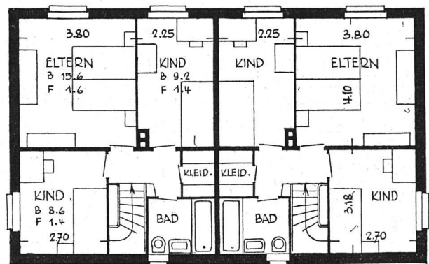
Obergeschoß
