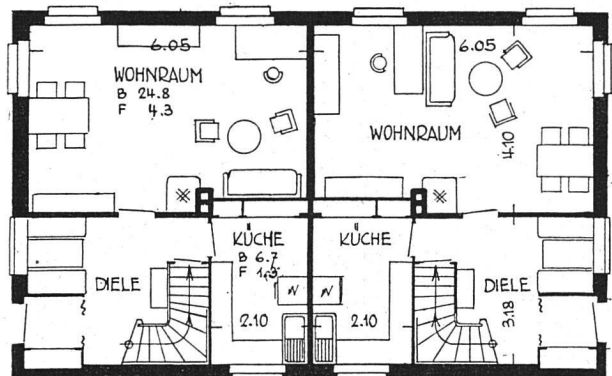
Erdgeschoß
