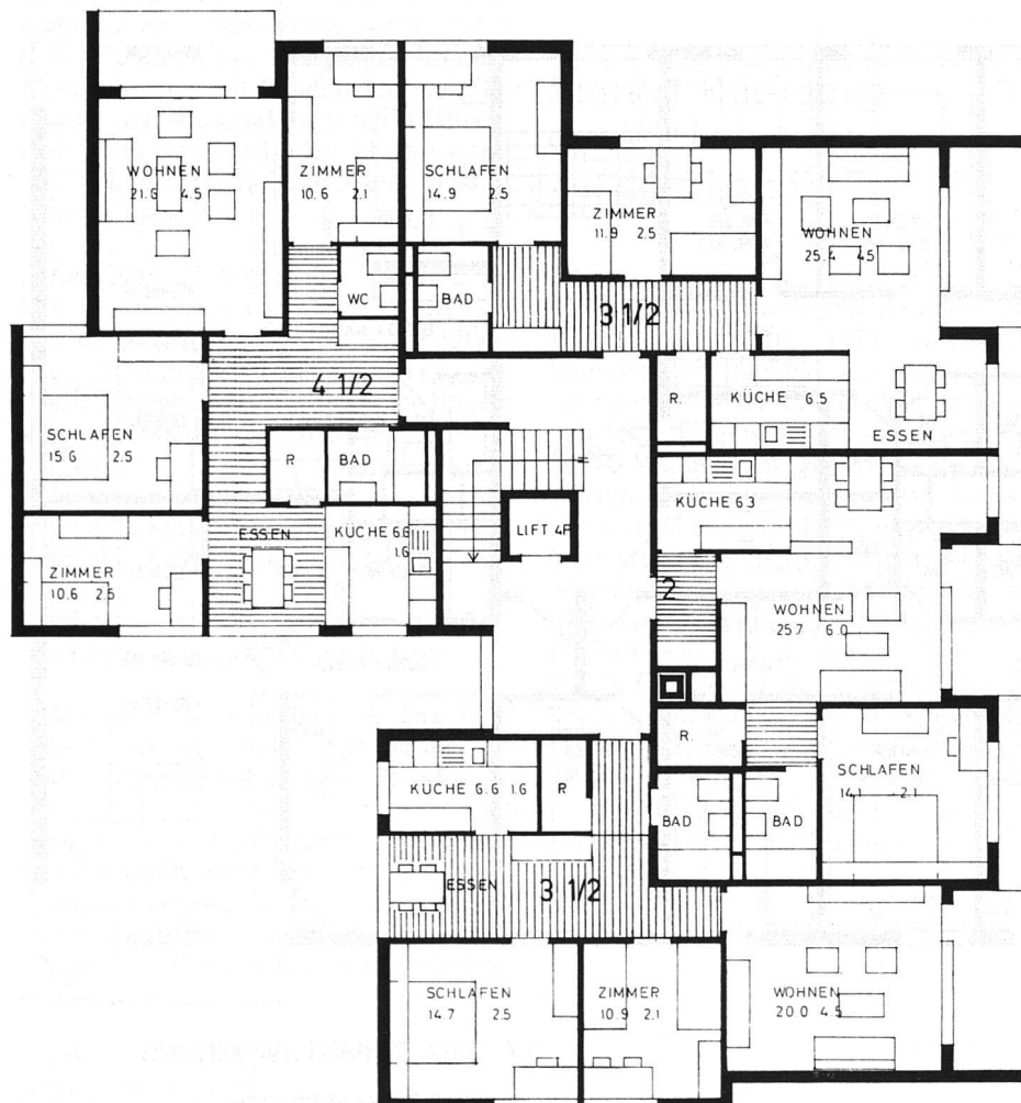
Oben: Grundriss aus der neuen Überbauung der Baugenossenschaft Pfäffikon.
