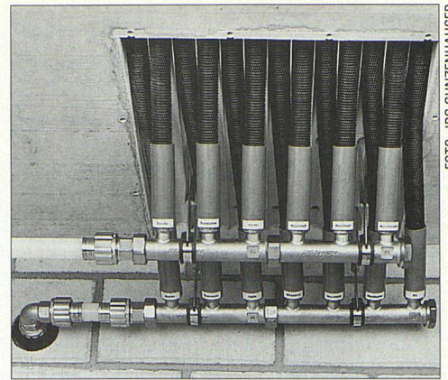
JRG Sanipex-System. Kalt- und Warmwasserverteiler unter der Kellerdecke
