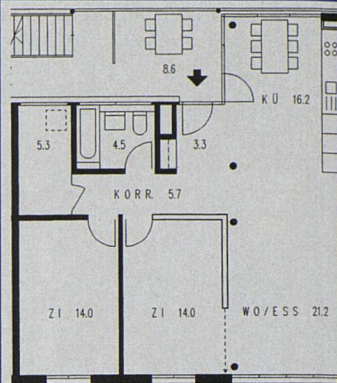
3 1/2-Zimmer-Wohnung Zwängiwiese
