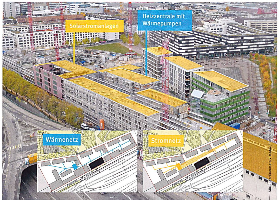
Im Quartier Erlenmatt Ost betreibt die ADEV seit dem Herbst 2017 eine der grössten Solarstrom-Eigenverbrauchsgemeinschaften der Schweiz.
