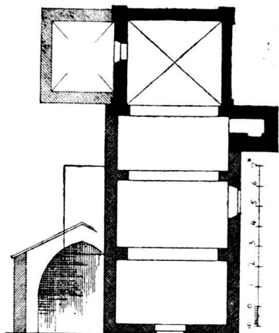
Fig. 121. Pfarrkirche S. Stefano in Miglieglia.
