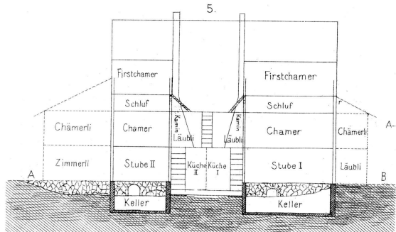
Längendurchschnitt 1:200
