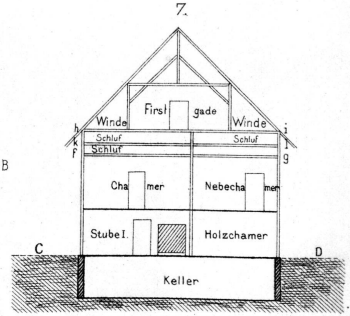
Querdurchschnitt 1:200
