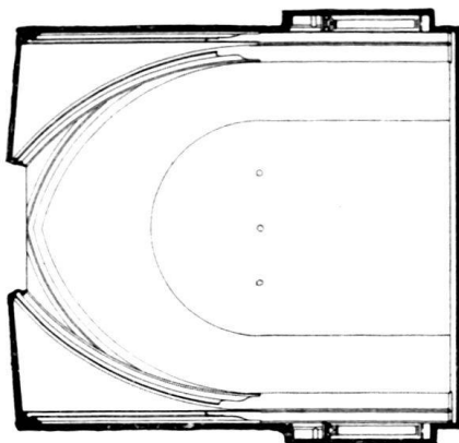
COUPE B-B
