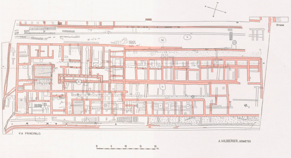
Abb. 1. Übersichtplan mit den Resten sämtlicher Bauperioden. Rot = Steinbauten
