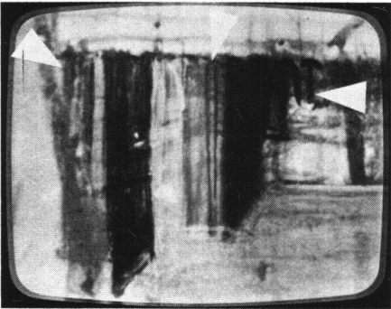
Abb. 29 Infrarot-Reflektogramm. Pfeiler des Helmhauses. Die ursprünglichen Holzpfähle, auf denen das Helmhaus stand, werden schwach sichtbar.
