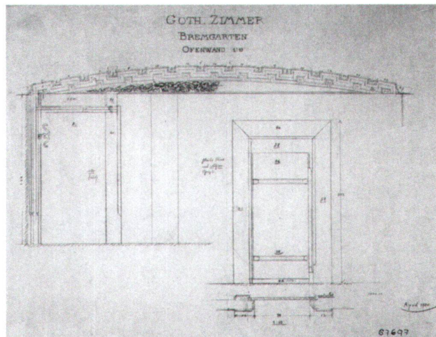
Abb. 41 Gotisches Zimmer, Bremgarten, Ofenwand, anonym, April 1900. Aufriss im Massstab 1:10. Zürich, Schweizerisches Landesmuseum. Inv. Nr. BS 1923.29–33.
