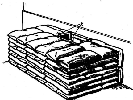
Abb. 8. Ausgebauter Notausstieg.
