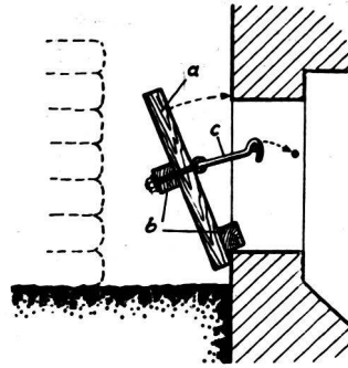
Abb. 6. Notausstieg.
