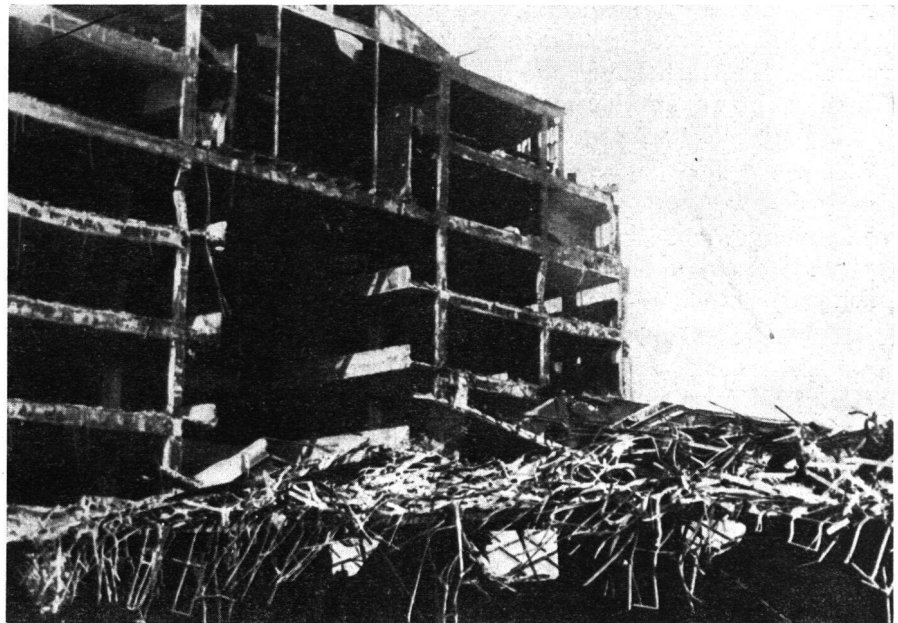
Abb. 16. Wirkung eines Volltreffers auf ein Eisenbetongebäude. Ein Volltreffer grössten Kalibers hat diesen Eisenbetonbau längs der Dilatationsfuge entzweierte. Am stehengebliebenen Teil sind nur zwei Säulen eingeknickt. Der Beton hat sich vom Eisen völlig getrennt. Die Bügel für die Schubsicherungen sind im Vordergrund deutlich erkennbar und so sauber vom Beton gelöst, als wären sie nie mit ihm verbunden gewesen. Dies legt die Vermutung nahe, dass beim Eisenbeton infolge verschiedener Schwingungszahl von Beton und Eisen die Verbundwirkung sich auflöste. Die Drähte, die vom abgeschnittenen Teil herunterhängen, sind elektrische Leitungsdrähte.
