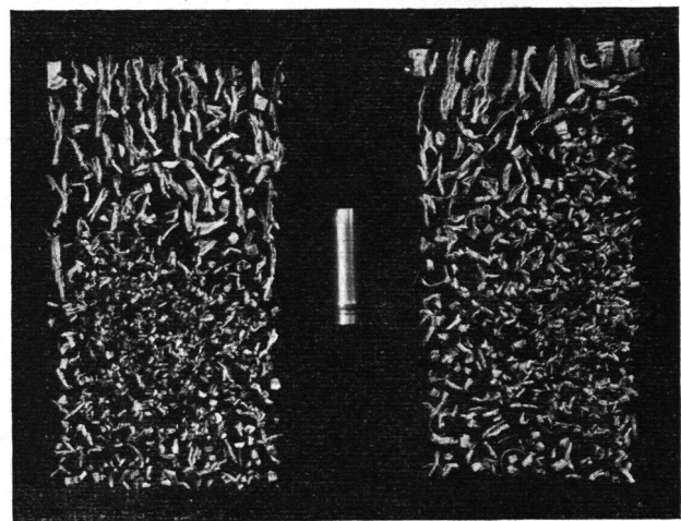
11,5 g Pentaerythrittetranitrat : 854 Splitter
