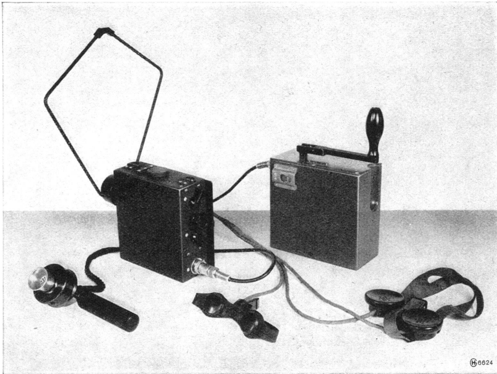
3. Hasler-UKW-Zweikanal-Kleingerät, Typ 1944
