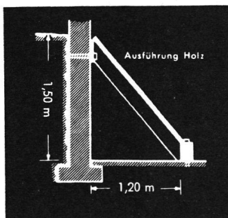
Schrägdachunterschlupf.
