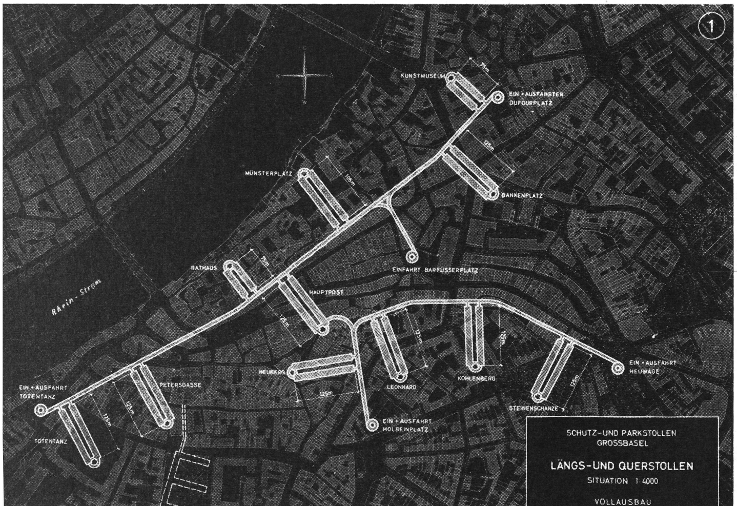
Unterirdischer Park- und Schutzstollen in Basel. Geplant ist die Erstellung von mehreren Verkehrstunnels mit elf seitlich eingebauten (mehrstöckigen) Querstollen unter dem Stadtkern, 25 m unter der Erde. — Zweck: Schaffung neuer Parkflächen für rund 2800 Motorfahrzeuge und Schutzräume für rund 35 000 Personen sowie die Unterbringung des Rettungs- und Bergungsdienstes; ausserdem können noch wertvolle Sammlungen der Museen und Vorräte aller Art dort untergebracht werden. Ferner sind noch Verbindungsstollen mit den Luftschutzkellern angrenzender Liegenschaften (als Notausgang) vorgesehen.
