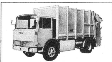
2) FBW: L 35 U Kehrriechtswagen Motor: FBW - CUA (130 PS) Getriebe: Allison MT-41 (Automat)
