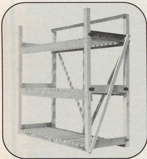
Schutzraumliege BK 86
