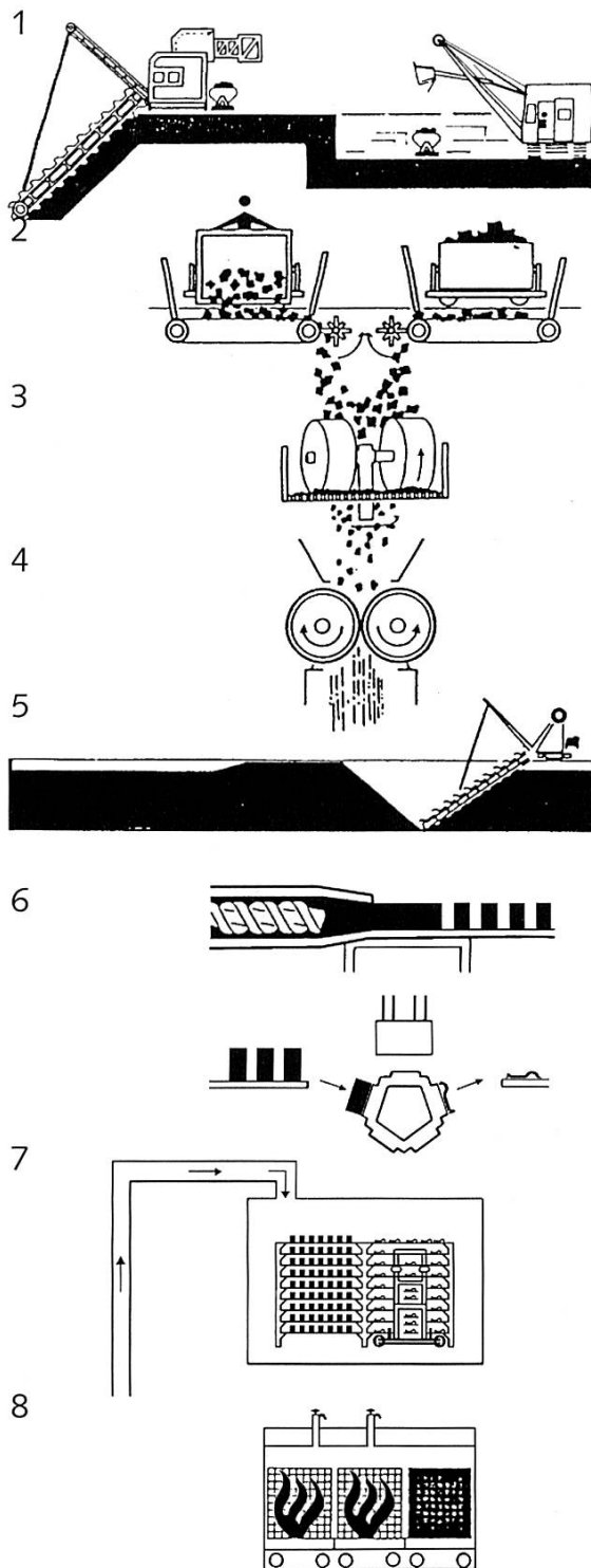
Abb. 2 Acht Stadien des mecha- nisierten Herstellungs- prozesses von Dachziegeln.
