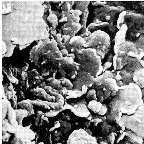
Abb. 3 Tonplättchen des ungebrannten Dachziegels; 1760-mal vergrössert.
