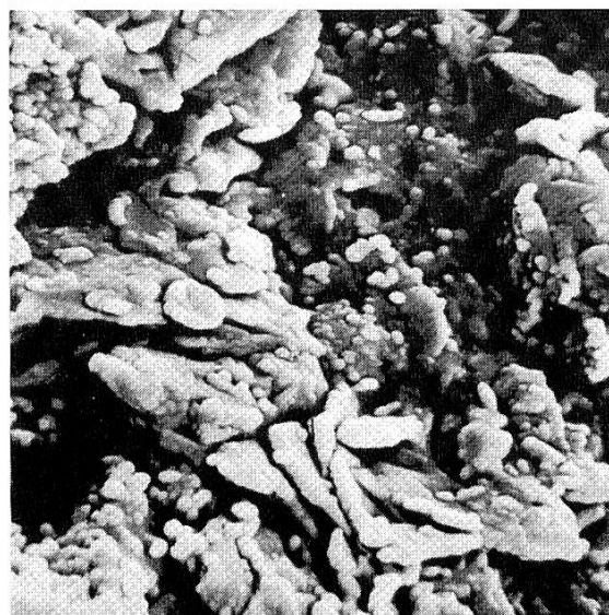
Abb. 4 Beginnende Bildung von neuen Mineralphasen ab 850 °C; 4800-mal vergrössert.
