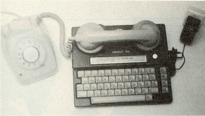
Das Schreibtelefon Telescrit 1005 ermöglicht das Lesen von Mitteilungen.
