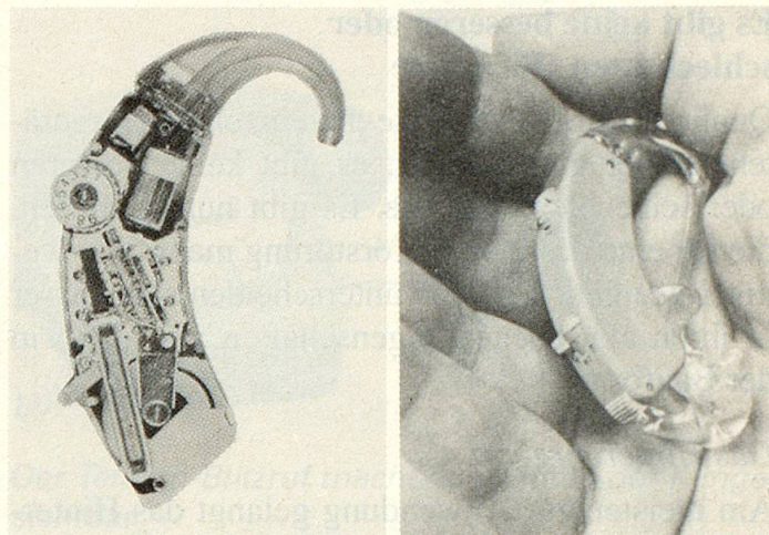
Modernste Technik auf kleinstem Raum, hier im Hinterohrgerät. Fotos: Wider-Hörgeräte AG
