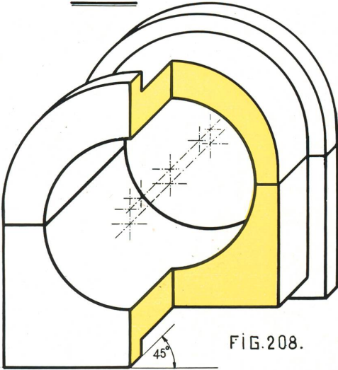
HORIZONTALE u. VERTIKALE MASSE 1:1, SCHRÄGE 1:2.
