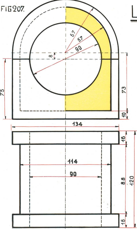
HORIZONTALE u. VERTIKALE MASSE 1:1, SCHRÄGE 1:2.
