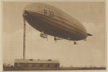
Das englische Luftschiff R 33 am Ankerplatz in Falmouth. Zwischen den beiden Gondeln ist das aufblasbare Flugzeug ersichtlich.
