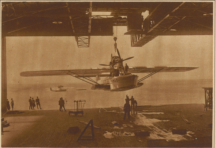
Ein neuer «Dornier Super Wal», der in Friedrichshafen gebaut wurde. Die Maschine soll beim künftigen Bau noch etwas vergrößert werden, so daß 60 Passagiere mit einer Geschwindigkeit von 180 km befördert werden können
