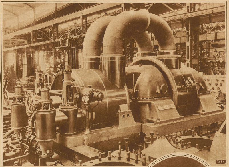
Eine neue zweigehäusige, 40000 P.S. Zoelly - Dampfturbine modernster Bauart, wie sie von der Firma Escher Wyß für das Straßburger Elektrizitätswerk geliefert wurde
