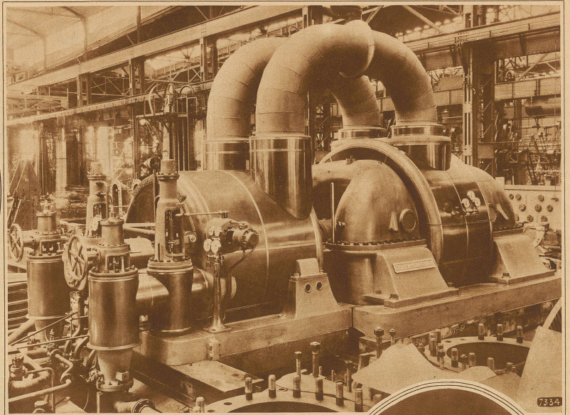
Eine neue zweigehäusige, 40000 P.S. Zoelly - Dampfturbine modernster Bauart, wie sie von der Firma Escher Wyl für das Straßburger Elektrizitätswerk geliefert wurde
