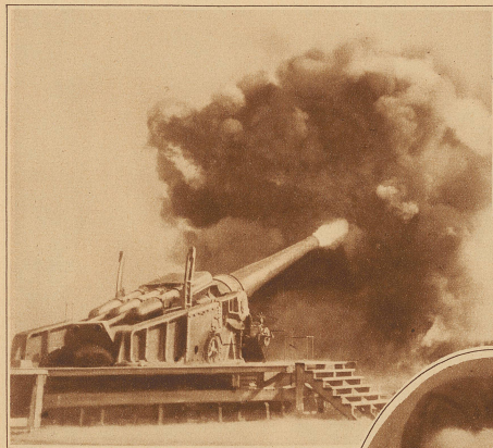
Abschuß eines neu gebauten 16 Zoll Langrohr-Geschützes auf dem Prüffeld von Aberdeen bei Washington. Es ist dies das größte Geschütz, das bis heute gebaut wurde
