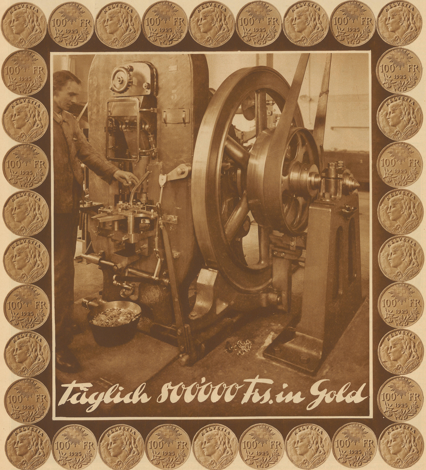
liefert diese Prägemaschine in der eidgenössischen Münzstätte in Bern
