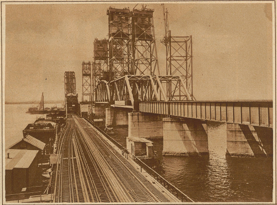
Das Mittelstück mit der Aufzugsvorrichtung
