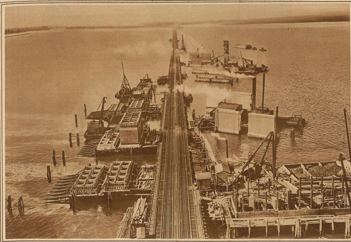
Teilsicht der Brücke während des Baues
